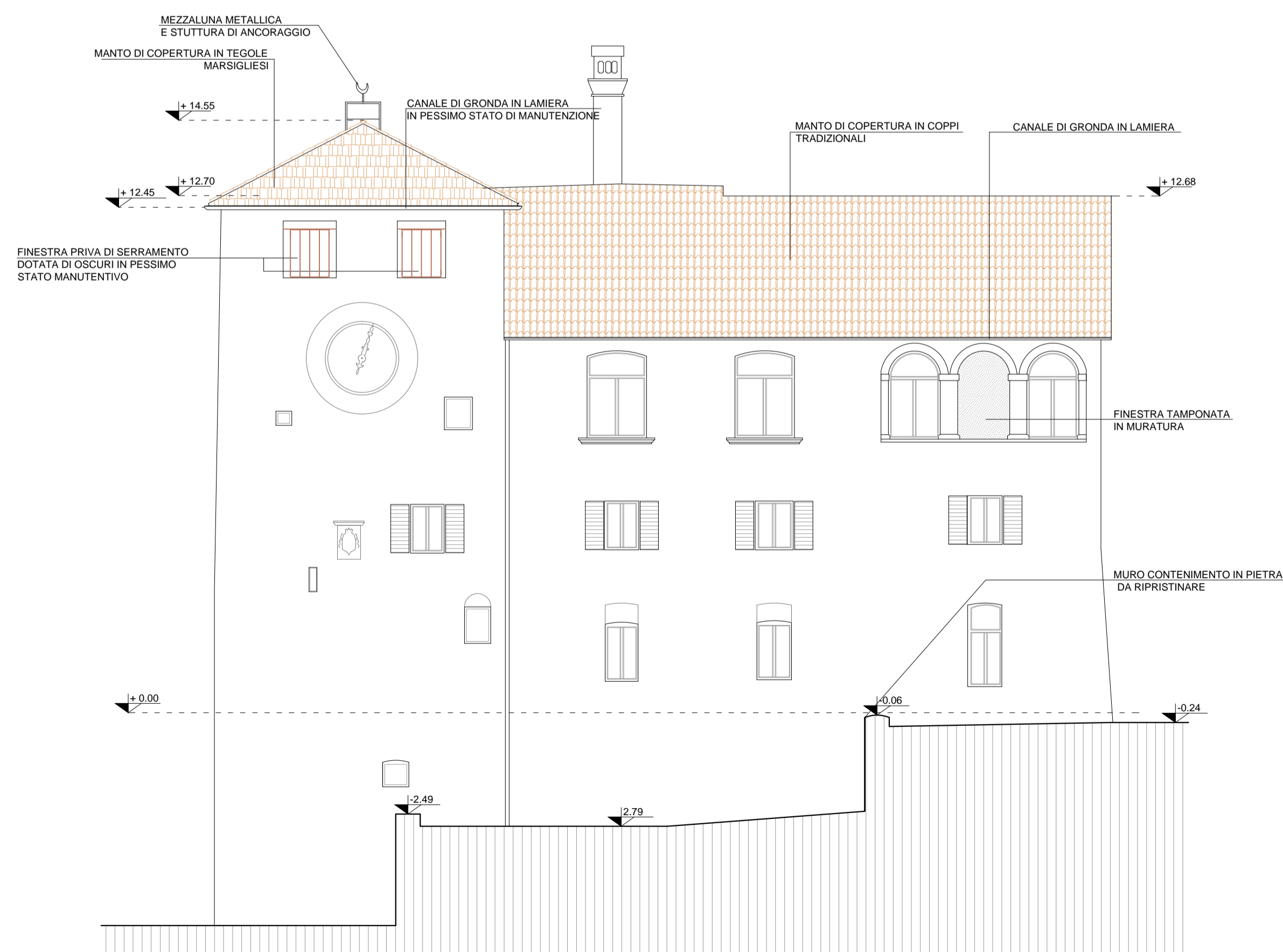
PROSPETTO SUD
