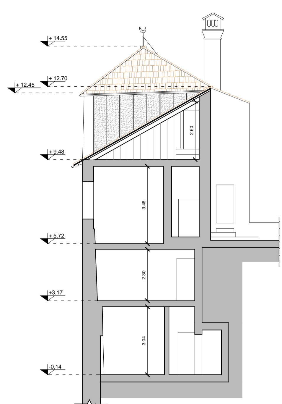
SEZIONE BB
