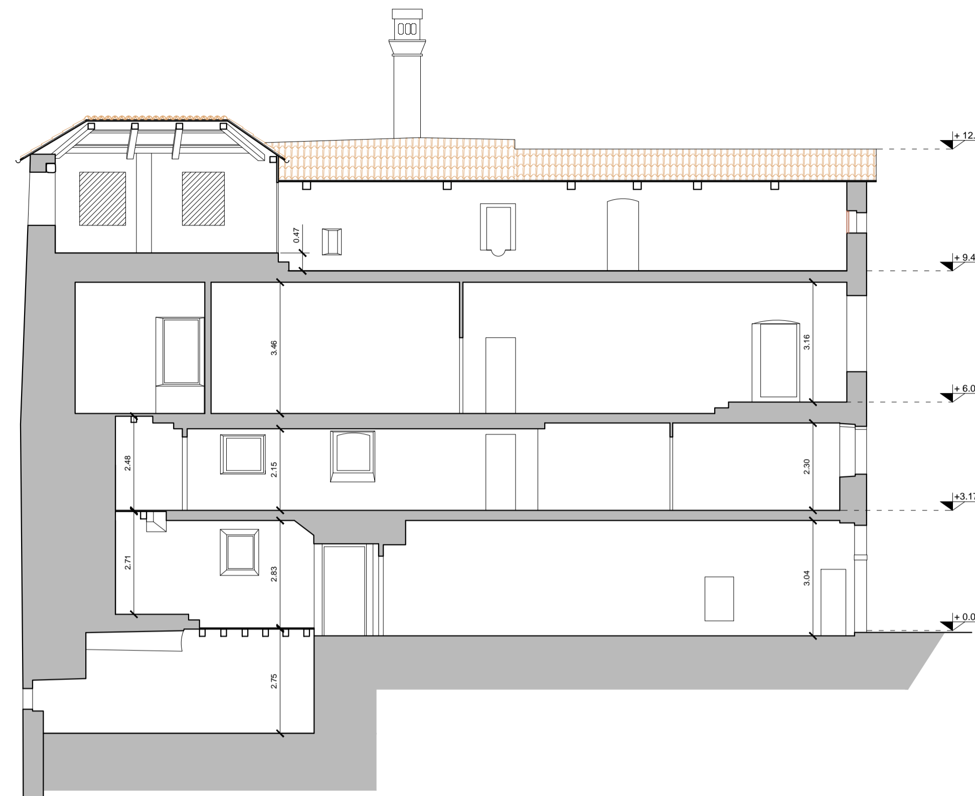
SEZIONE CC
