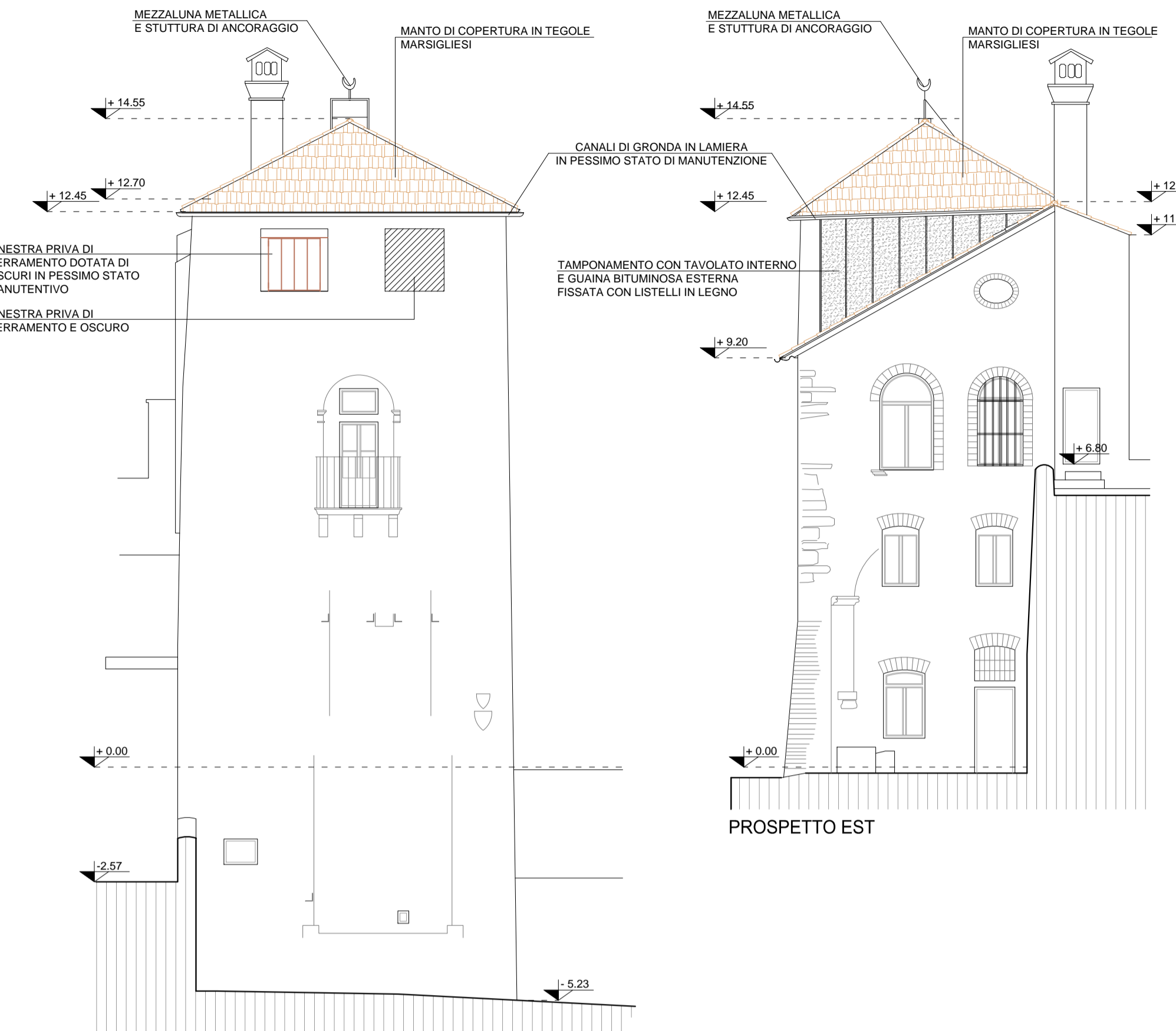
PROSPETTO OVEST
