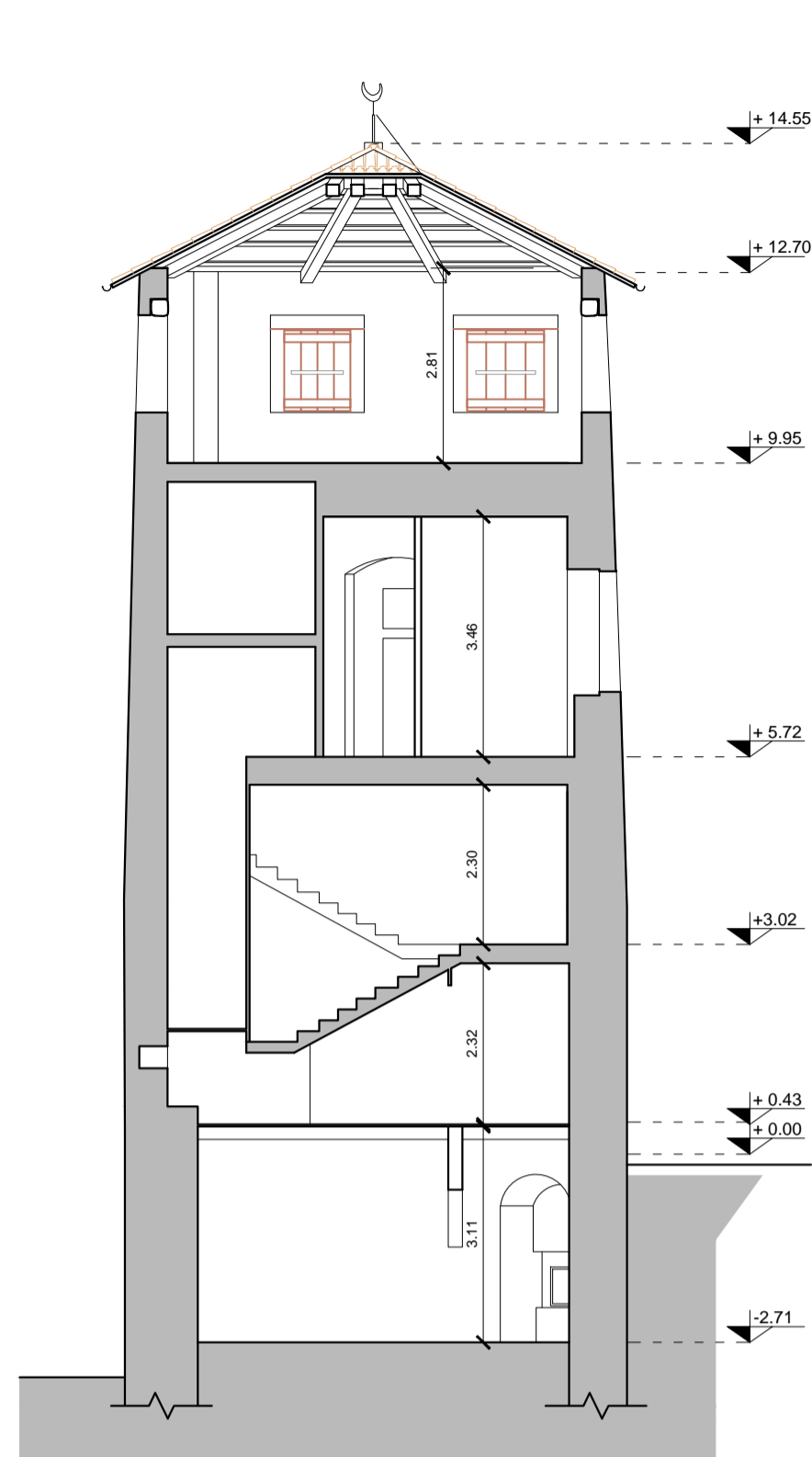
SEZIONE AA
