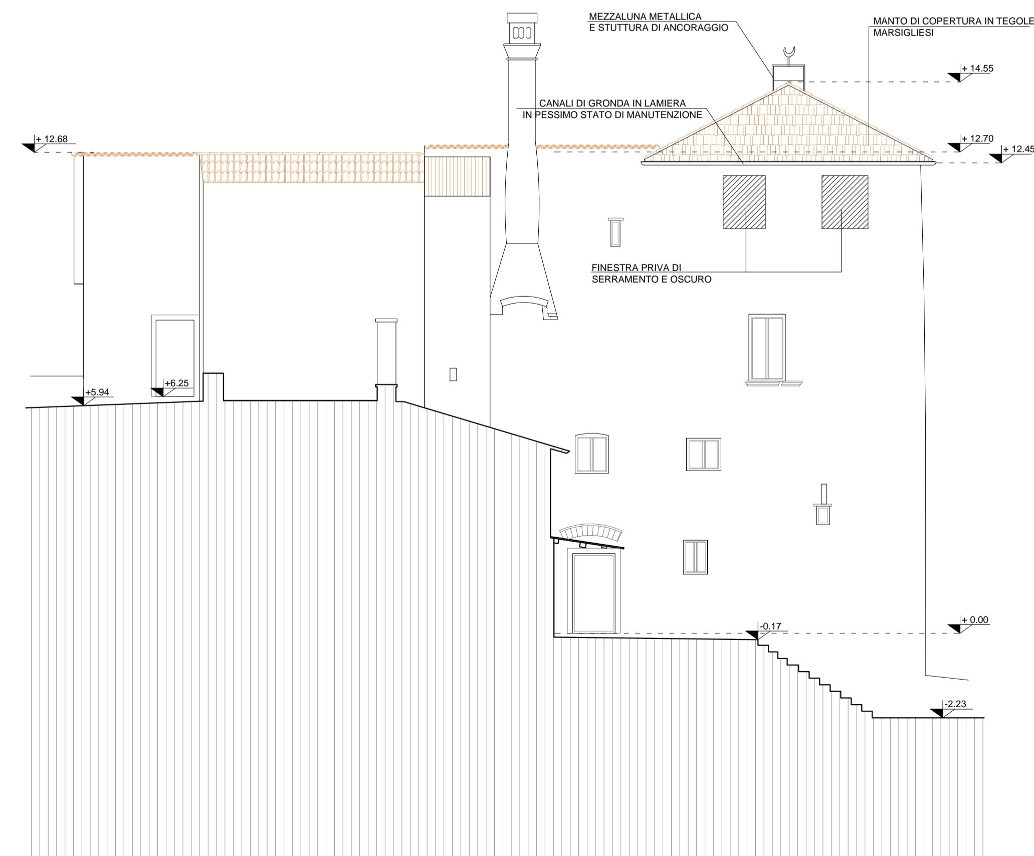
PROSPETTO NORD
