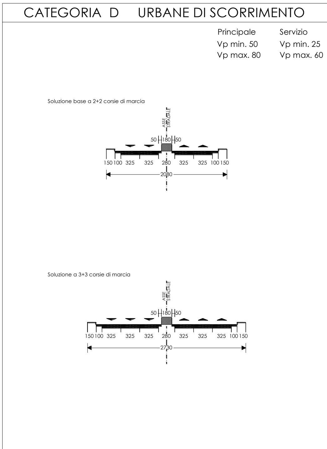
Figura 5-1 – Strada Urbana di Scorrimento - Sezione Tipo ("Norme funzionali e geometriche per la costruzione delle strade" (D.M. n.6792 del 5 novembre 2001)
