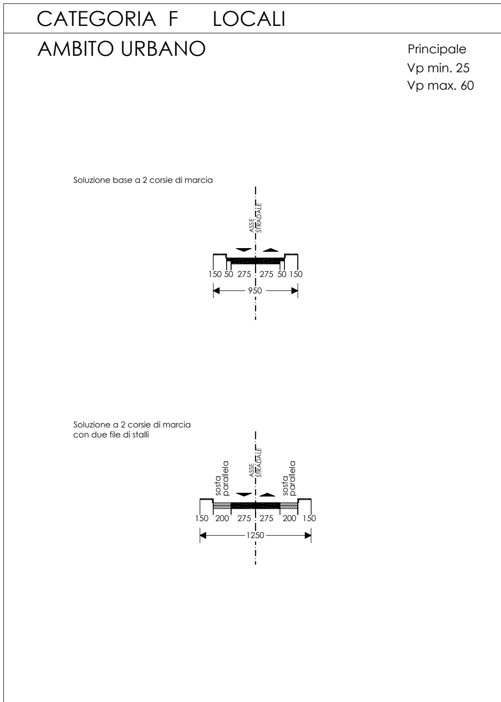
Figura 9-1 - Strada Urbana Locale - Sezione Tipo ("Norme funzionali e geometriche per la costruzione delle strade" (D.M. n.6792 del 5 novembre 2001)
