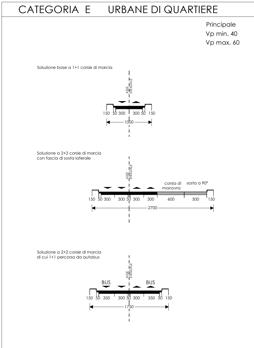
Figura 7-1 - Strada Urbana di Quartiere - Sezione Tipo ("Norme funzionali e geometriche per la costruzione delle strade" (D.M. n.6792 del 5 novembre 2001)
