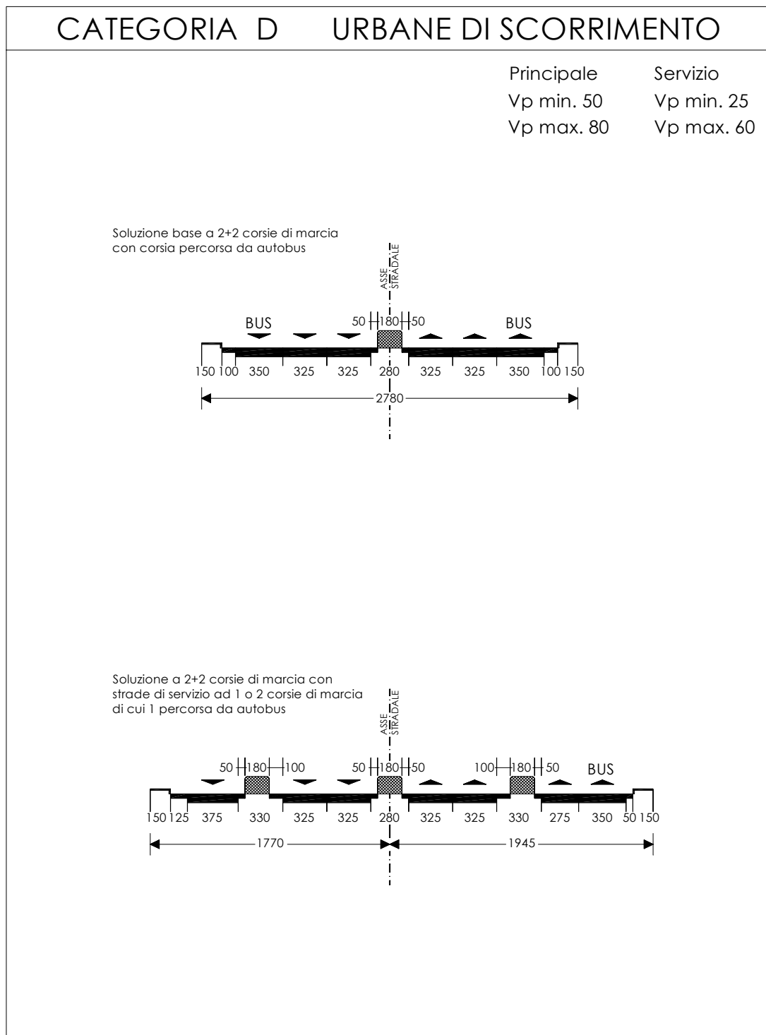
Figura 5-2- Strada Urbana di Scorrimento - Sezione Tipo ("Norme funzionali e geometriche per la costruzione delle strade" (D.M. n.6792 del 5 novembre 2001)
